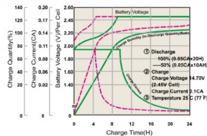
نمودار متحنی شارژ در حالت استفاده
